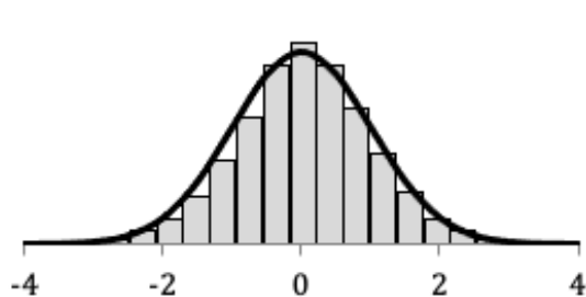
Abb. 2 Histogramm (Normalverteilung)
